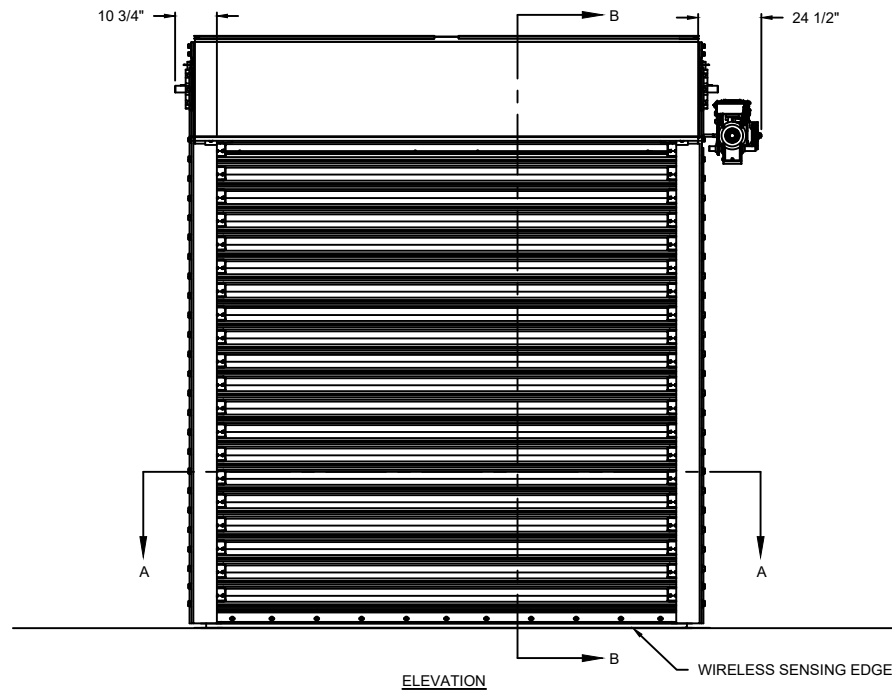
ELEVATION
