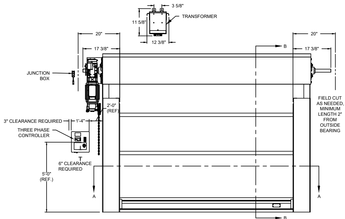
ELEVATION
