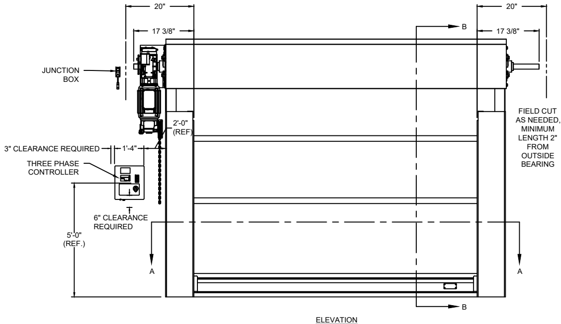
ELEVATION
