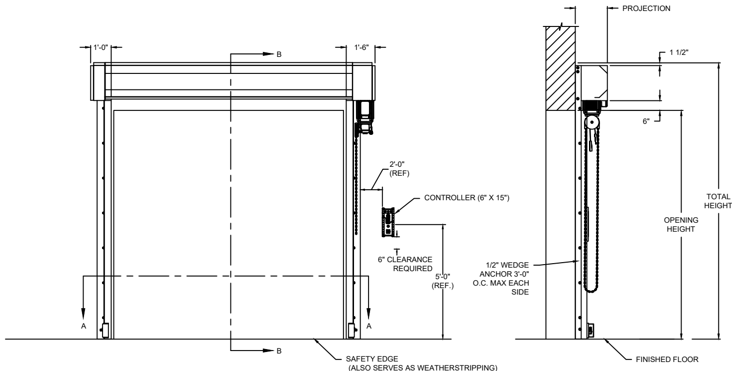
ELEVATION
